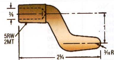
16-3838 CMW ® 3 CASTING
