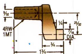
16-3873 CMW ® 3 CASTING
