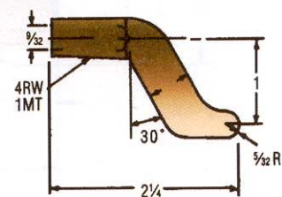
16-3835 CMW ® 3 CASTING
