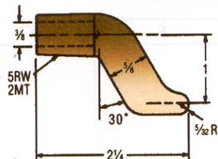
16-3836 CMW ® 3 CASTING
